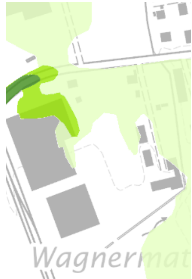
Abb. 9: Intensitätskarte HQ 100 (seltene Ereignisse), Naglerbach
